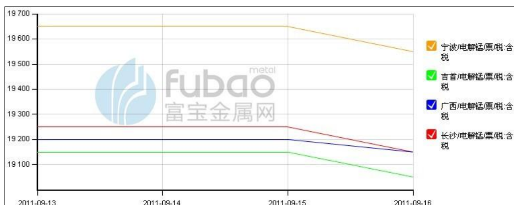
图 1: 全国主要地区电解锰价格走势 (2011.9.13-2011.9.16, 单位: 元/吨)
