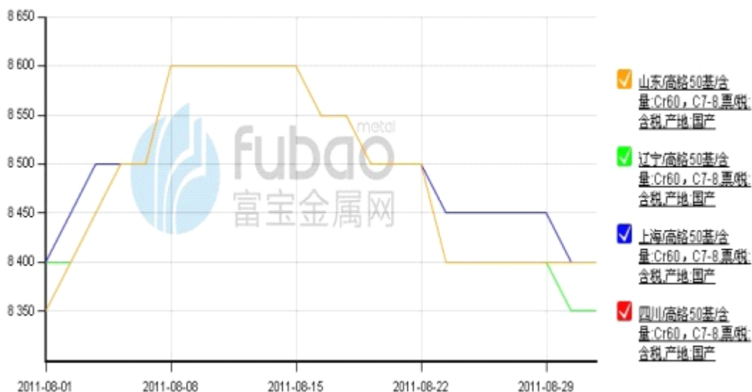
图2：7月四川、上海、辽宁、山东地区高碳铬铁价格走势 (元/基吨)
