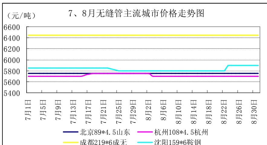
图 3: 7、8月无缝管市场主流城市价格对比图
