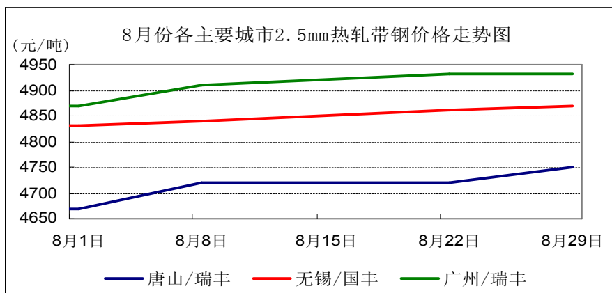
图 1: 8月国内主要市场 2.5mm 热轧带钢价格走势
